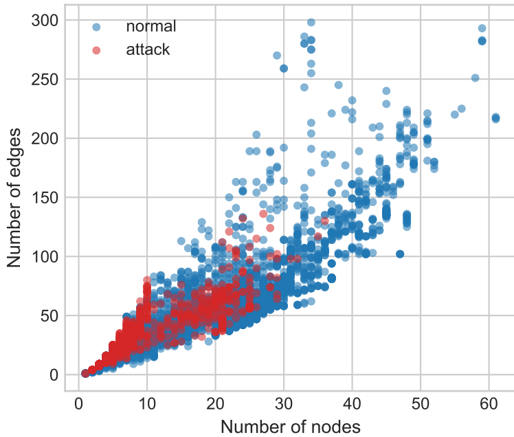
ADFA-LD
